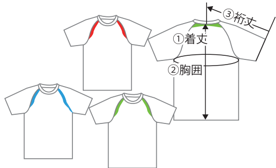
Tシャツ 出来上がり寸法
